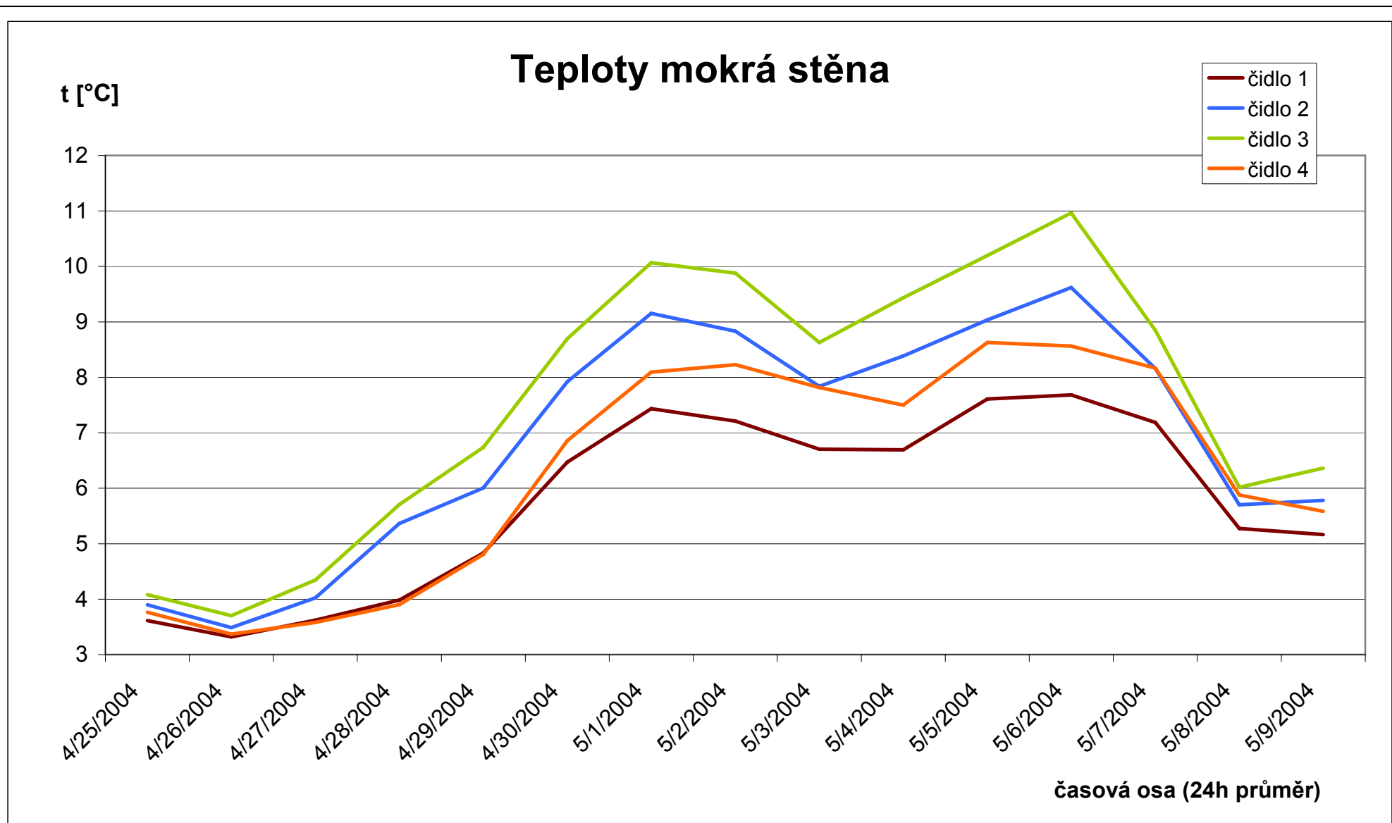
Graf 2. Teploty mokrá stěna. Hodnoty naměřené 4 teplotními čidly, umístěnými ve shodné výšce nad zemí a zdánlivě stejných abiotických podmínkách na mokré stěně, v časovém úseku od 25.4. do 9.5. 2004. Z grafu je patrné, že se průměrné teploty v některých dnech lišily i více než o 3°C. Pravděpodobně zde má vliv mikroklima jednotlivých míst.
