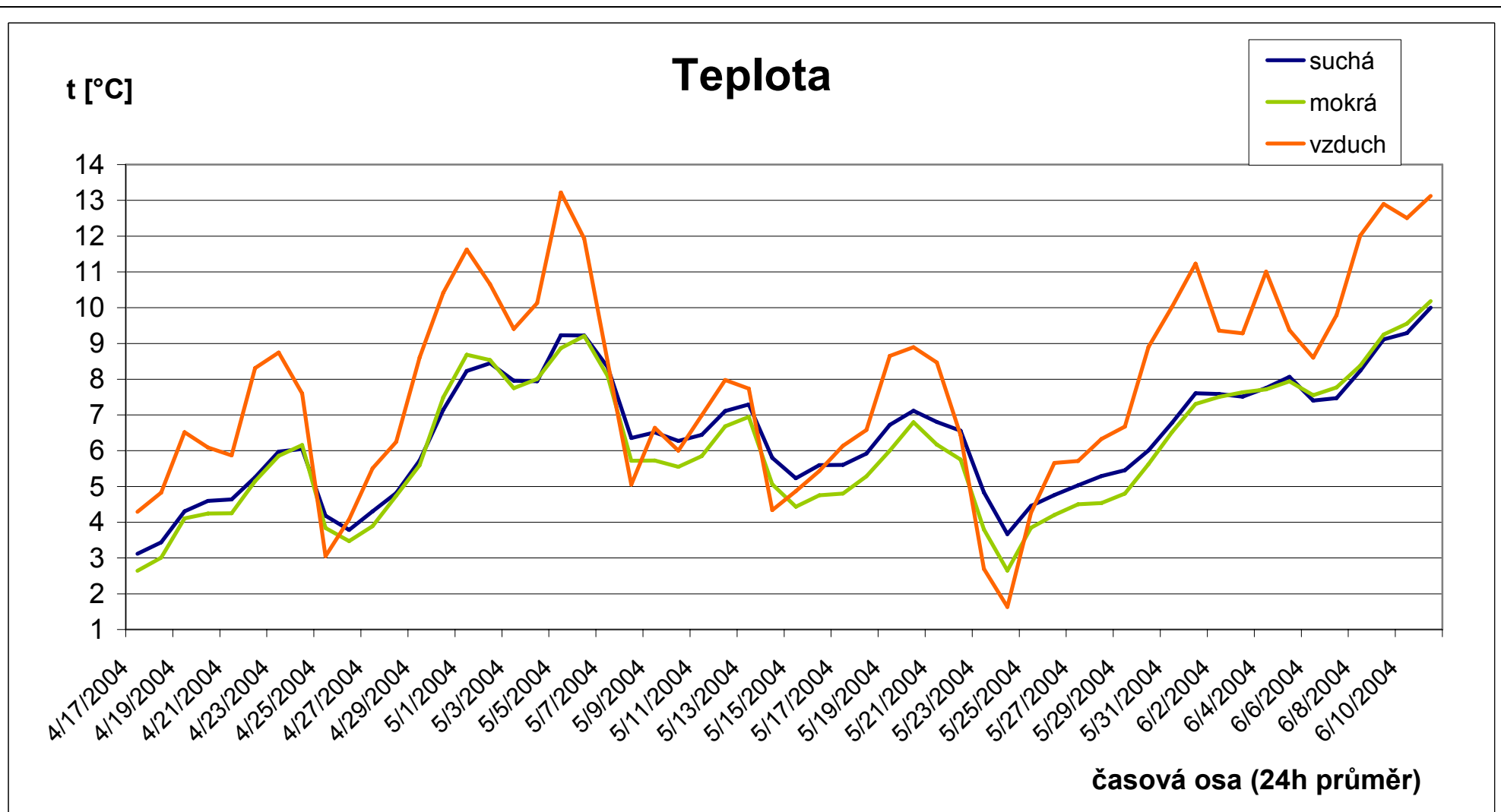
Graf 1. Teploty. Oranžová, nejvíce kolísající křivka přísluší teplotám vzduchu uprostřed rokle, modrá průměru 2 teplotních čidel na suché stěně a zelená průměru 4 čidel na mokré stěně. Křivky pro teploty povrchu protilehlých skalních stěn mají podobný průběh, na mokré stěně byly dle původního předpokladu naměřeny o něco nižší teploty (maximální rozdíl v sledovaném období je v denním průměru cca 1,5°C). Na křivce pro suchou stěnu nejsou v porovnání s křivkou pro stěnu mokrou patrné výraznější výkyvy ve směru maximálních hodnot, což by poukazovalo na její větší prohřívání během slunečných dnů. Křivka pro teploty vzduchu, měřené uprostřed rokle se od křivek teplot skalního povrchu zřetelně liší, dosahuje extrémních hodnot grafu.
